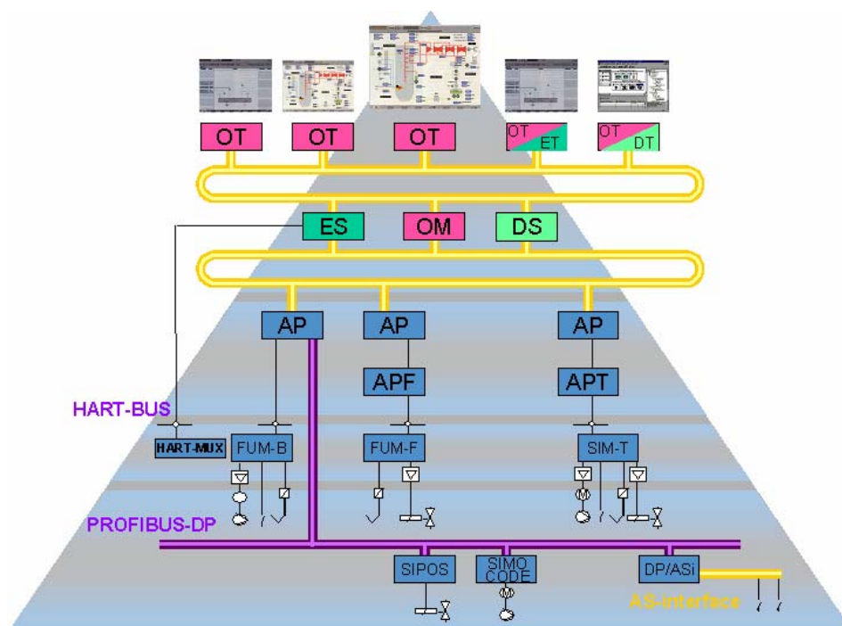
图 1 系统配置图
